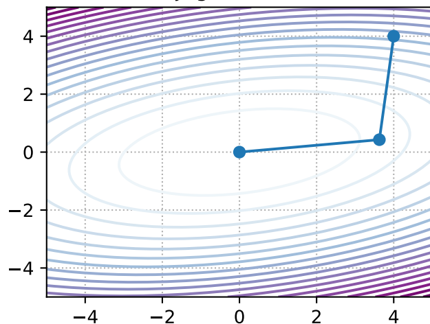
Conjugate Gradient
